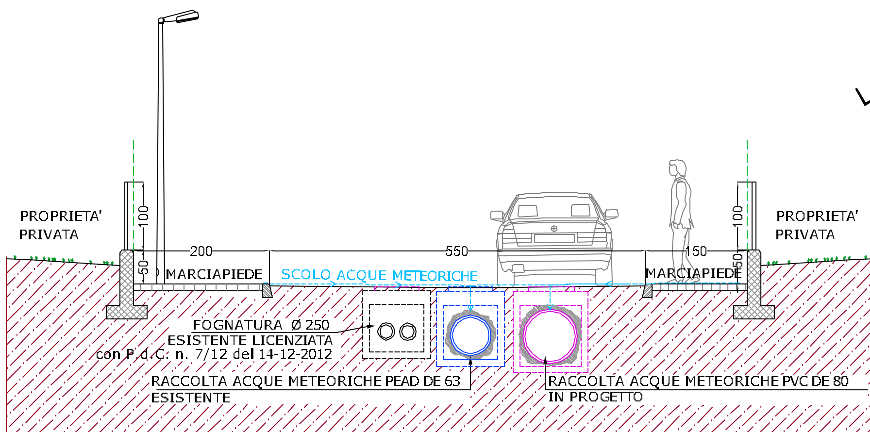
SEZIONE TIPO X/X SEZIONE TRASVERSALE DELLA STRADA INTERNA PRIVATA Scala 1:50
