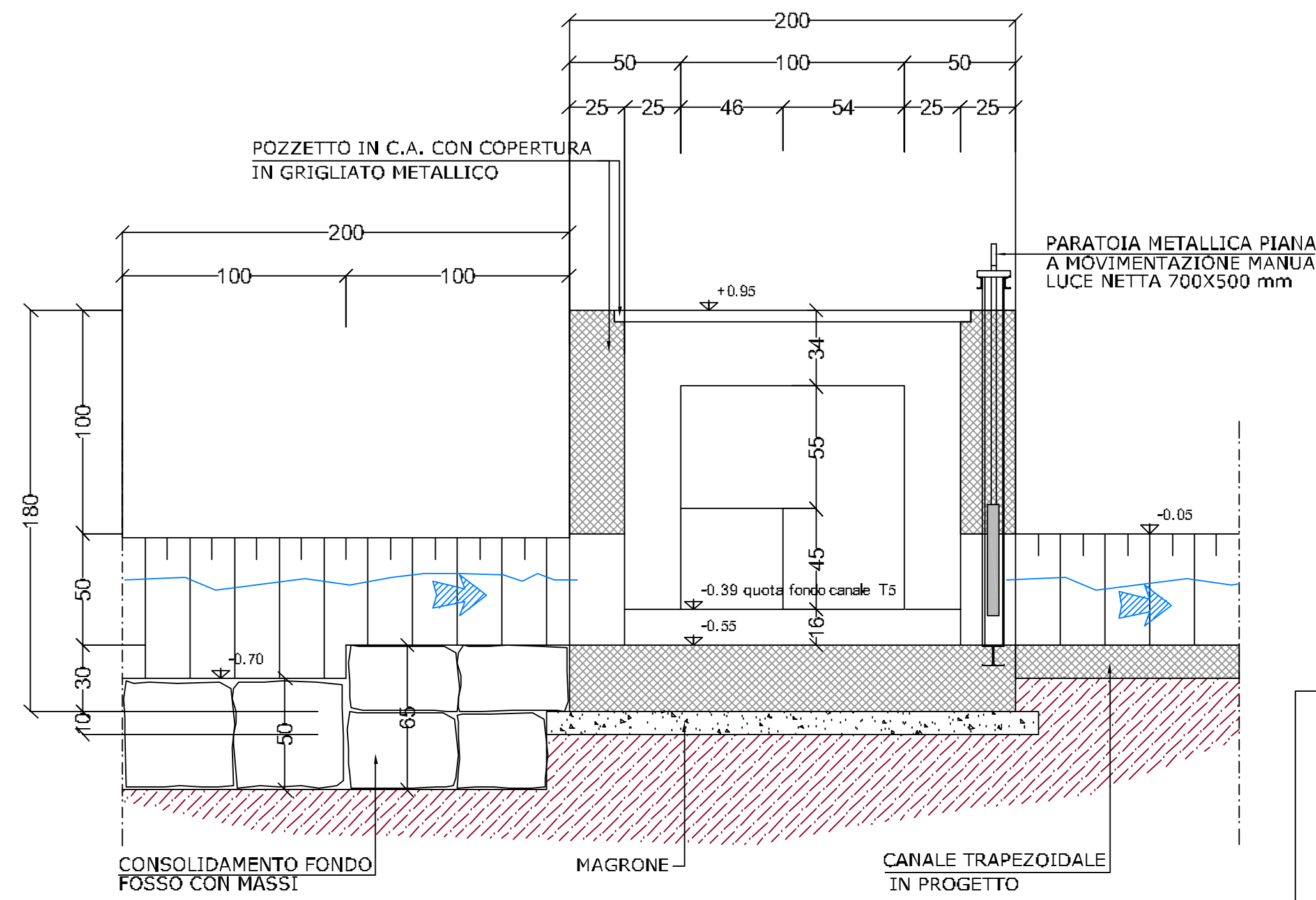
PARTICOLARE 1 POZZETTO PARTITORE - SEZIONE Scala 1:20
