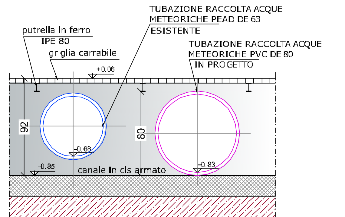
PARTICOLARE 3 INNESTO TUBAZIONI NEL CANALE APERTO Scala 1:20
