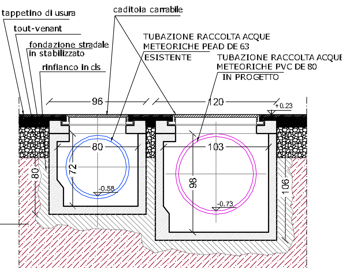
PARTICOLARE 4 POZZETTI CARRABILI - SEZIONE TIPO Scala 1:20
