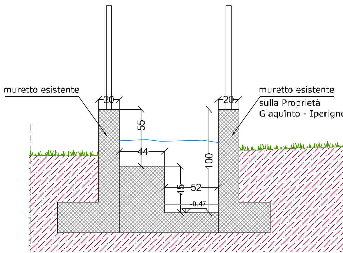
PARTICOLARE 2 CANALE GRIGLIATO APERTO IN CLS Scala 1:20
