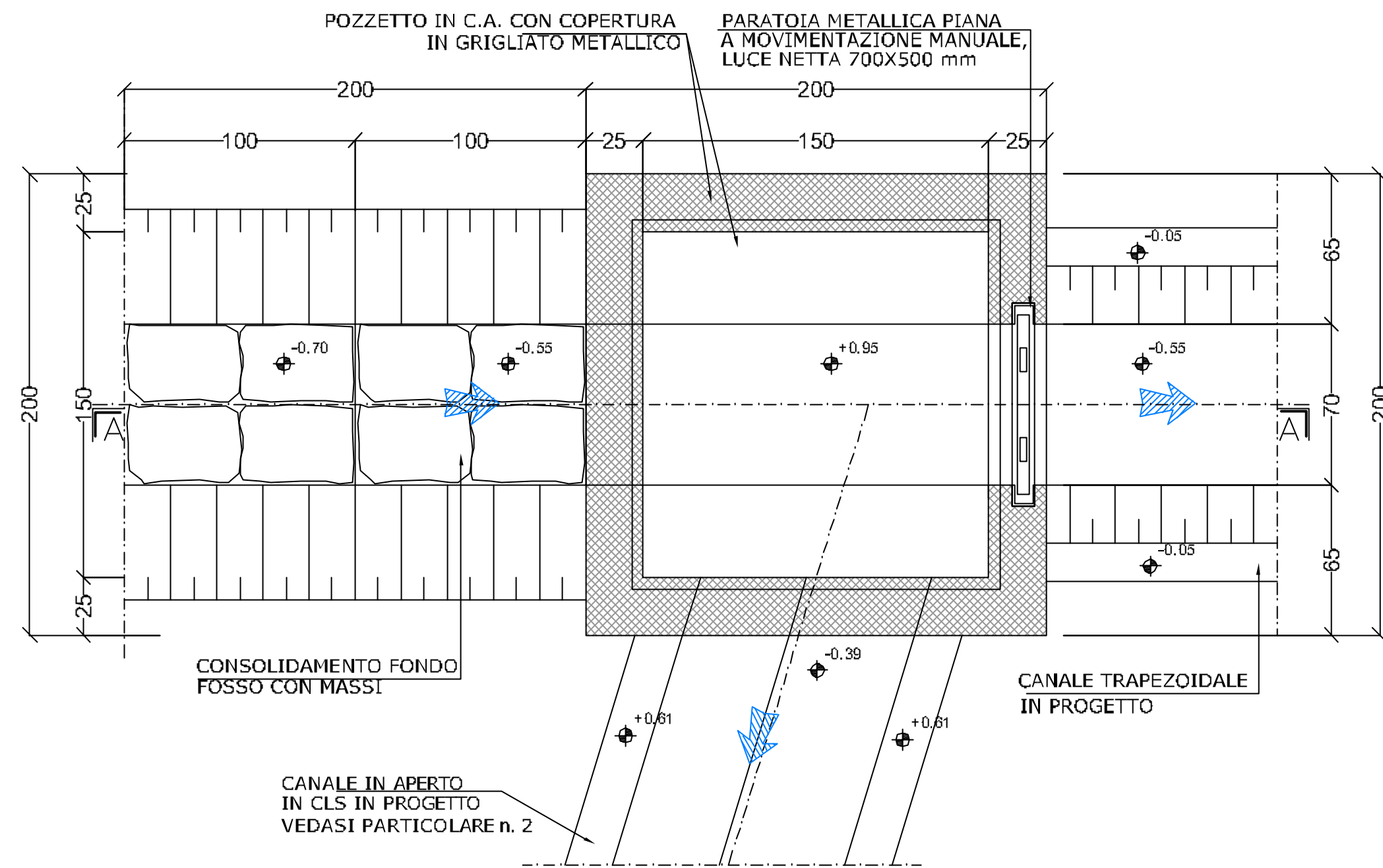
PARTICOLARE 1 POZZETTO PARTITORE - PIANTA Scala 1:20
