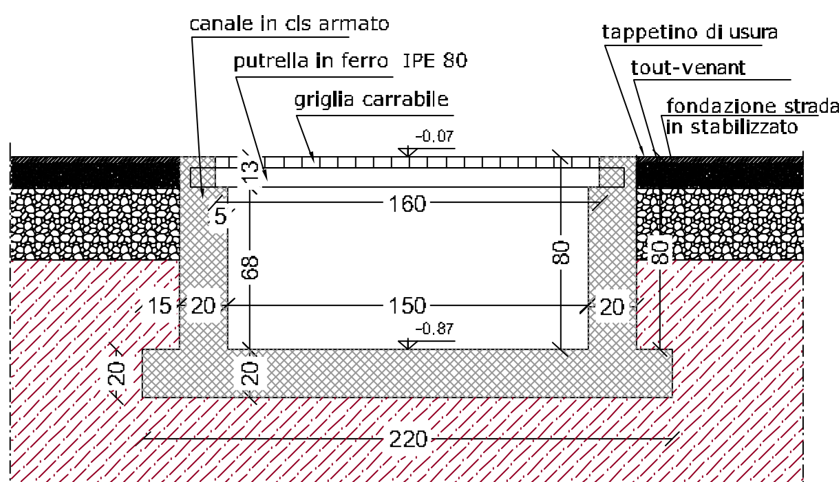
PARTICOLARE 5 CANALE GRIGLIATO IN CLS - SEZIONE TIPO Scala 1:20
