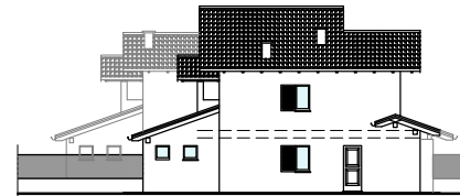
PROSPETTO NORD-OVEST lotto 3
