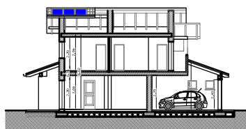
SEZIONE C - C
