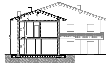
SEZIONE B - B
